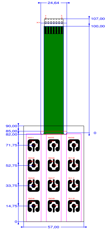
Frontansicht der Kontaktpads:
